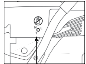
Stationairschroef carburateur
